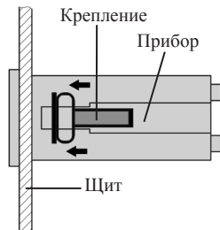
Рис. 2 – Установка прибора
